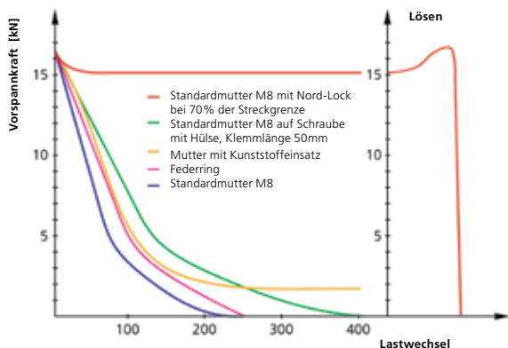
Abb. 1: Das Junker-Diagramm zeigt die einzigartige Sicherungswirkung der Nord-Lock Sicherungsscheiben. Es treten nur geringe Vorspannkraftverluste durch normale Setzungs Vorgänge zwischen den Trennfugen und dem Gewinde auf. Die Keilsicherungsfunktion wird durch den deutlichen Anstieg der Klemmkraft während des Lösevorgangs bestätigt. Herkömmliche Sicherungselemente zeigen unter Vibration keine Sicherungswirkung.
